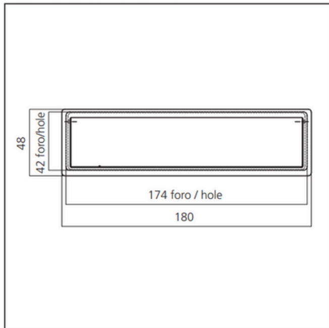
sezione / section
