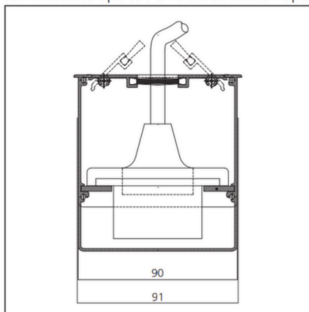
sez. incassato aperto / embedded section open
