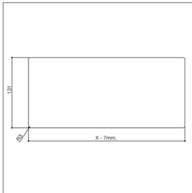
dim. foro hole template
