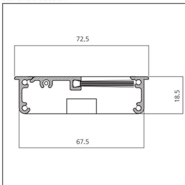
sezione / section
