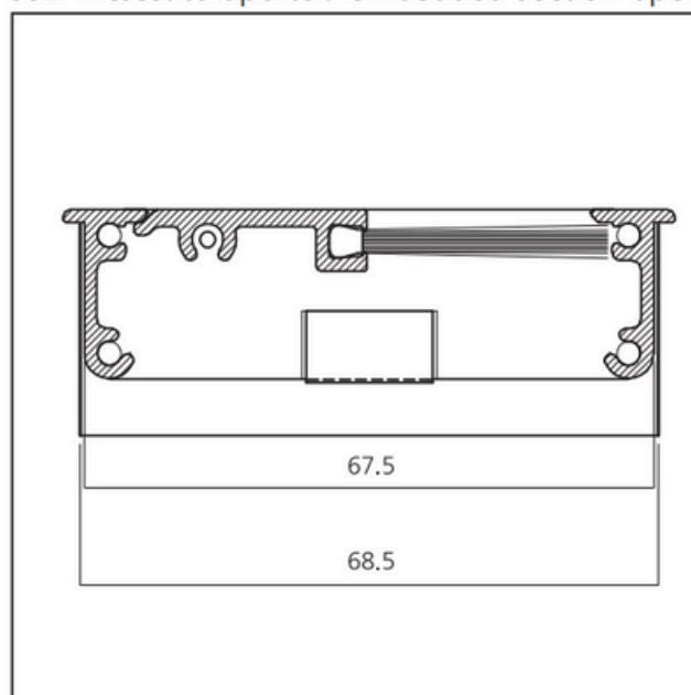
sez. incassato aperto / embedded section open
