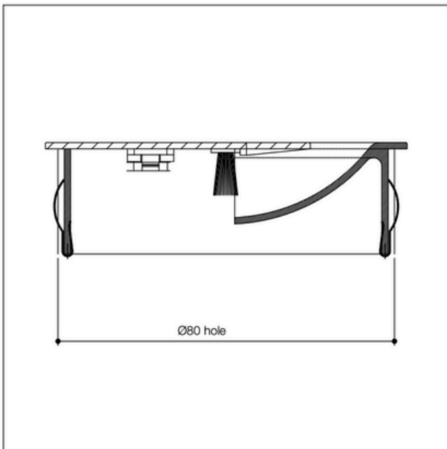
sezione section
