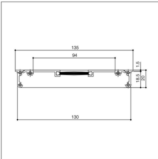
sezione section
