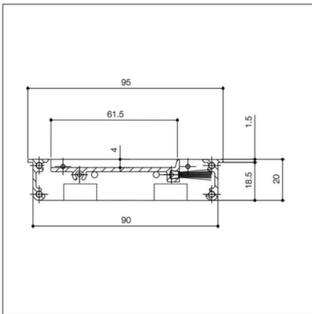
sezione section
