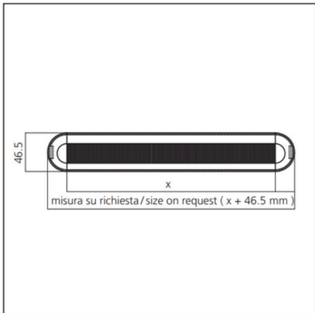
sezione / section
