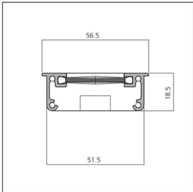
sezione / section
